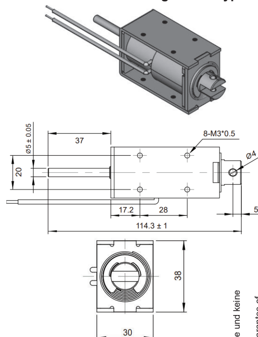
Drückende Ausführung / Push Type
