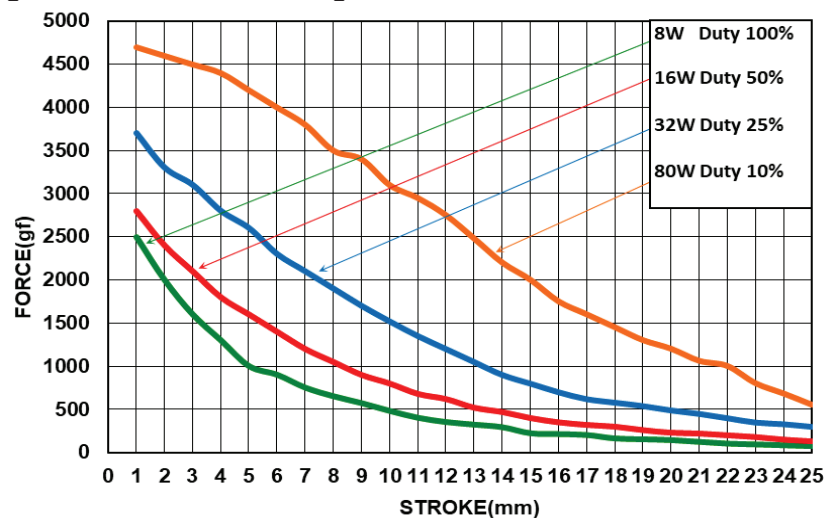
Kraft-Wege-Diagramm / Stroke-Force-Diagram
